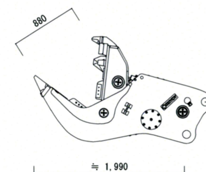
小割機仕様
