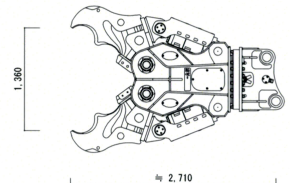
クラッシャー仕様
