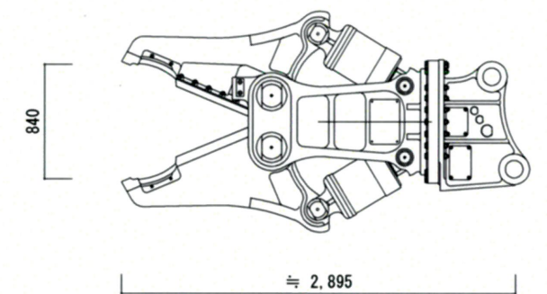
カッター仕様
